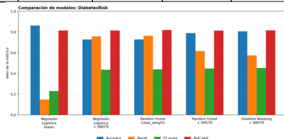
Figura 2. Comparación de métricas entre los 5 modelos entrenados
